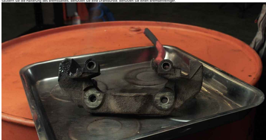
17 Säubern Sie die Halterung des Bremssattels. Benutzen Sie eine Drahtbürste. Benutzen Sie einen Bremsenreiniger.
