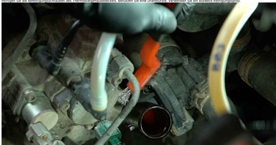
12 Schrauben Sie die Befestigungsschrauben des Thermostatgehäusedeckels ab. Verwenden Sie ein T25-Torx-Bit. Verwenden Sie eine Kardangeln-Steckschlüsselverlängerung. Verwenden Sie einen Ratschenschlüssel.
