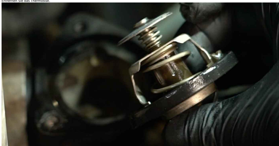
16 Reinigen Sie den Montagesitz des Thermostatgehäusedeckels. Verwenden Sie ein Allzweck-Reinigungsspray.
