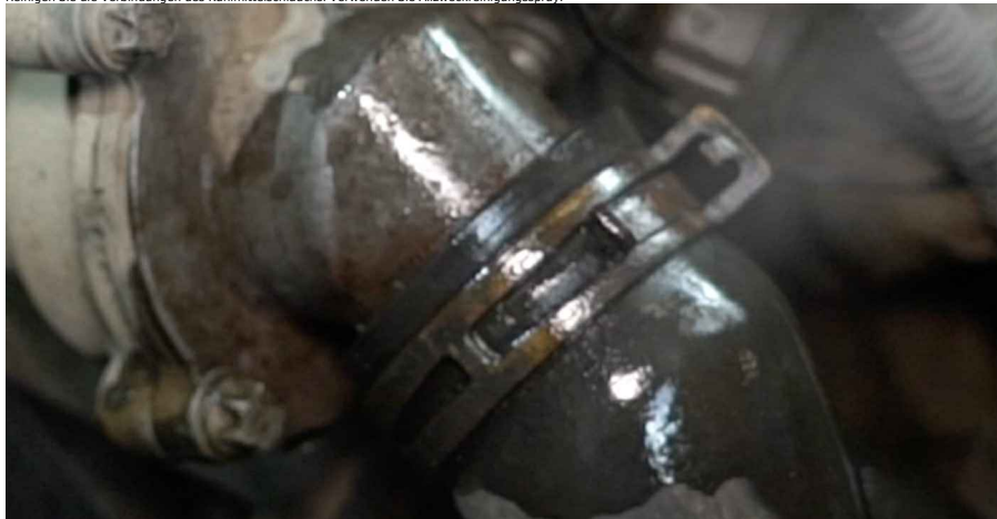
16 Lösen Sie die Klemmen der Kühlmittelschläuche. Verwenden Sie eine Clic-R-Kragenzange.
